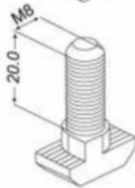
Parafuso "T" M8 p/ perfil 40/45
